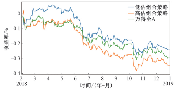
图 2 区间累计收益率
