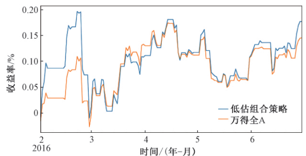
图 4 2016 年上半年累计收益率
