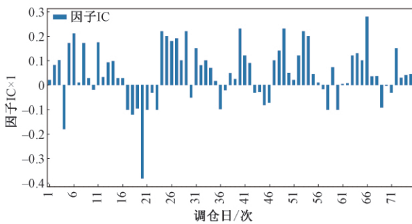
图 1 各期因子 IC 值
