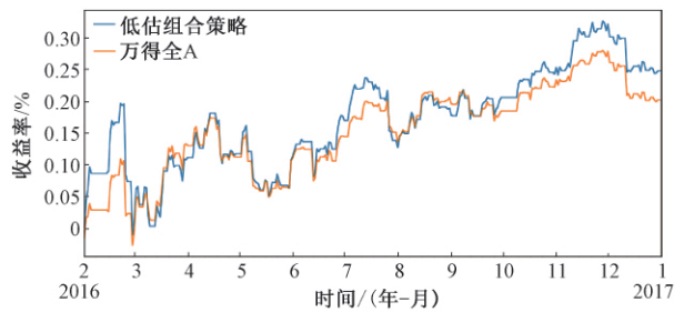
图 3 2016 年全年累计收益率
